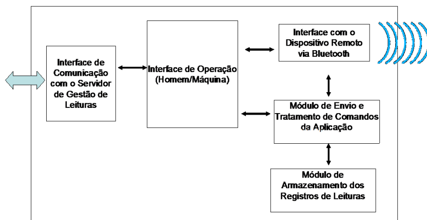
Figura 8 – Diagrama de Blocos do Firmware do Bluetooth
