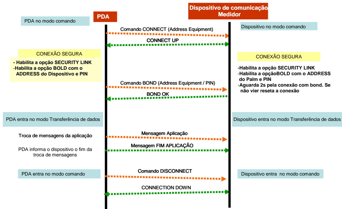
Figura 4 – Enlace de Comunicação do Bloco “Tratamento da Comunicação Bluetooth”
