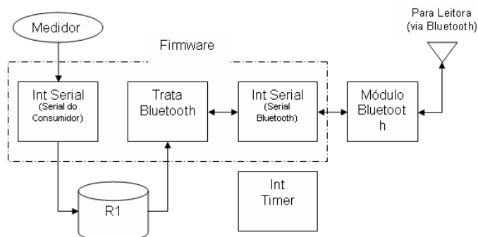
Figura 7 – Diagrama de Blocos do Firmware do Bluetooth
