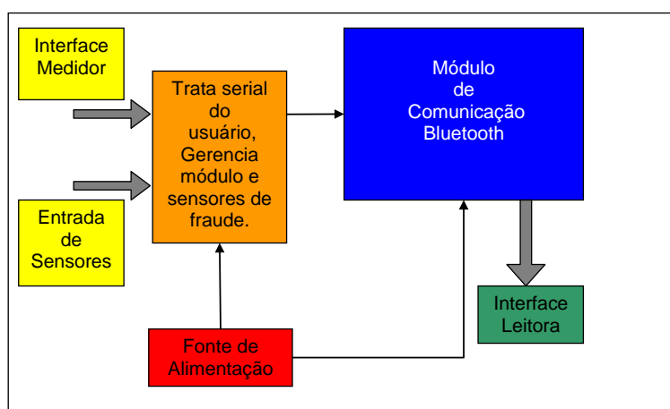
Figura 2 – Diagrama de Blocos do Dispositivo de Comunicação
