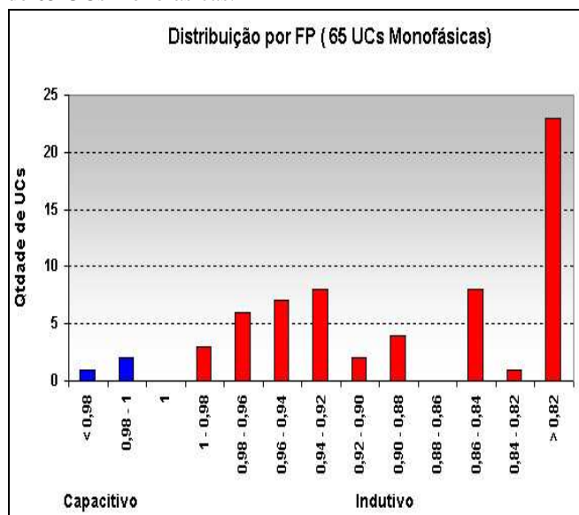
Figura 13. Distribuição por Tipo de Consumo Reativo
