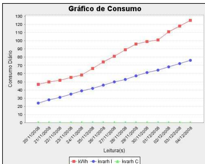
Figura 12. Consumo diário de uma UC no período de 15 dias
