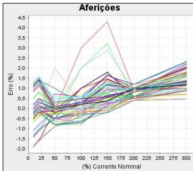
Figura 6. Qualidade da Aferição do Lote de medidores Monofásico correspondente à Situação 1.
